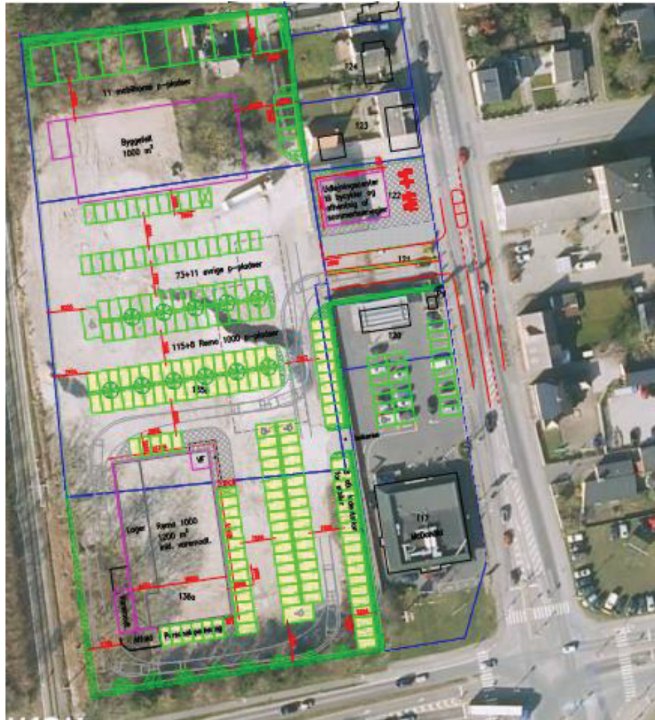
Figur 2. Principudformning af ny vejadgang til det kommende butiksområde på Århusvej.
