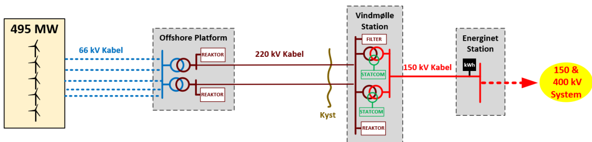
Figur 3-10 Elektrisk topologi
