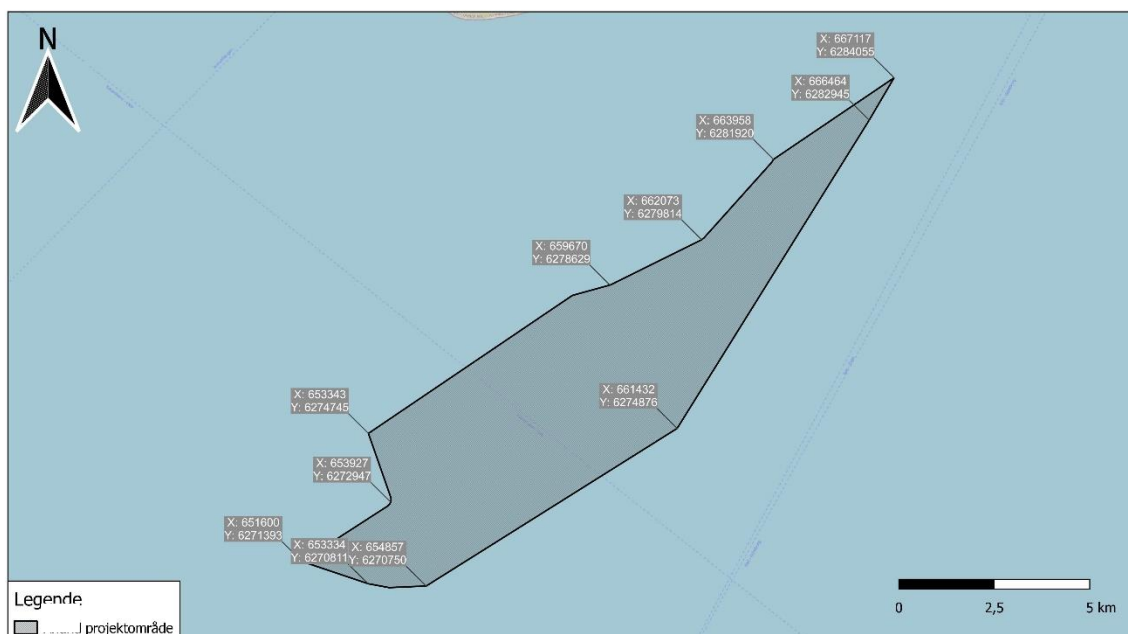
Figur 3-2 Layout med koordinater for Sønderbjerg Havvindmøllepark 2 projektområde.
