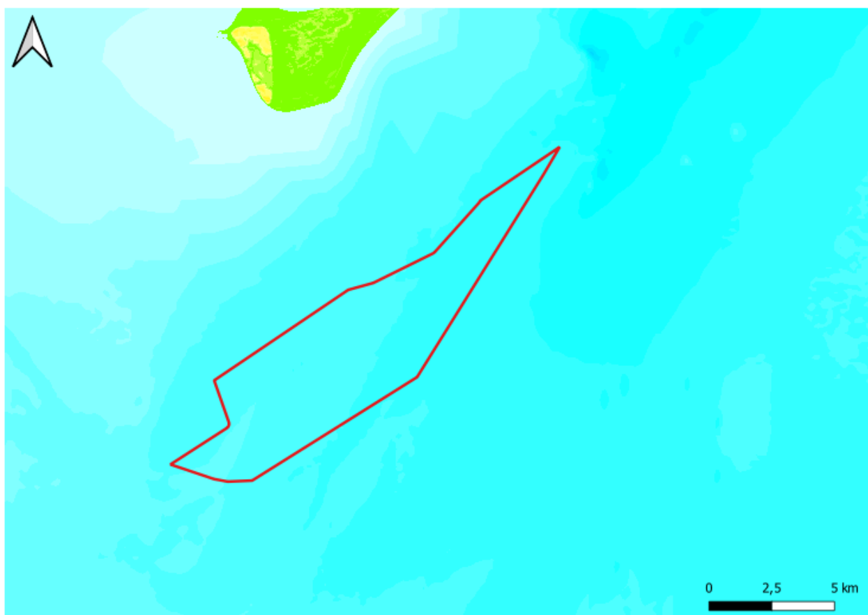
Figur 3-7 Batymetriske kort fra GEUS database. Sønderbjerg Havvindmøllepark 2 er afgrænset med røde linjer (nord for ligger Anholt).
