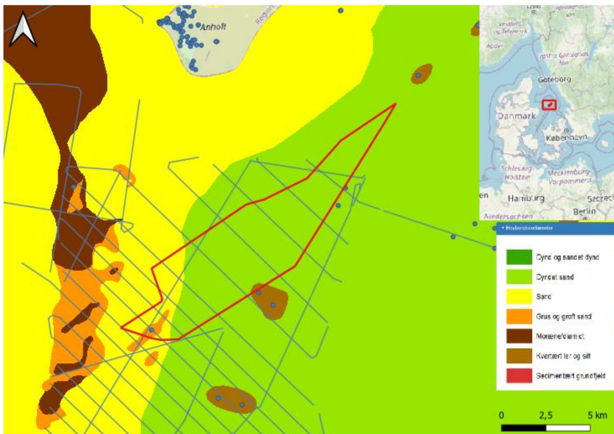
Figur 3-3 Havbundssedimentkort fra GEUS med borer (blå cirkler) og geofysiske surveys (blå linjer) Sønderbjerg Havvindmøllepark 2 området er markeret med rød outline.
