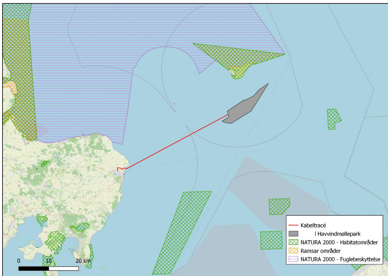
Figur 4-2 Forslag til kabeltracé og modtagerstation for Sønderbjerg Havvindmøllepark 2. Desuden ses nærmeste Natura 2000-områder og Ramsar-områder.
