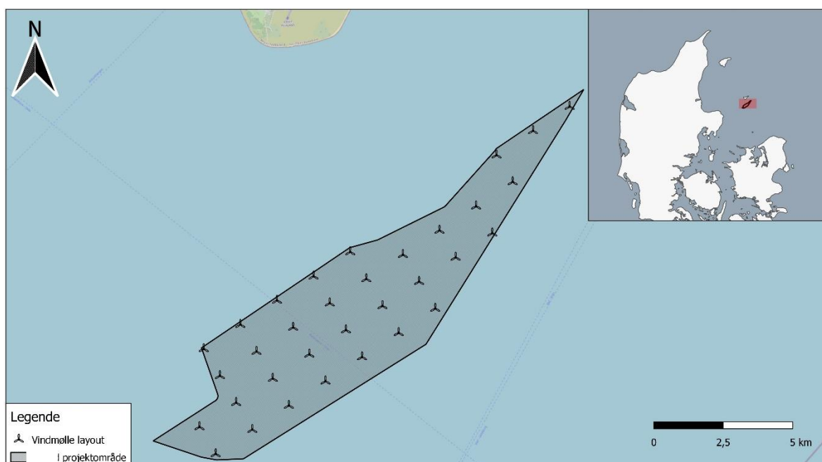
Figur 3-1 Layout af Sønderbjerg Havvindmøllepark 2
