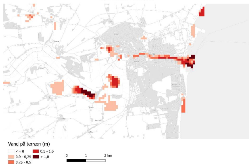
Figur 8.16 Vand på terræn ved en kote 3 stormflod i et døgn. Oversvømmelsen er især koncentrat omkring havnen og Grenåens bredder.
