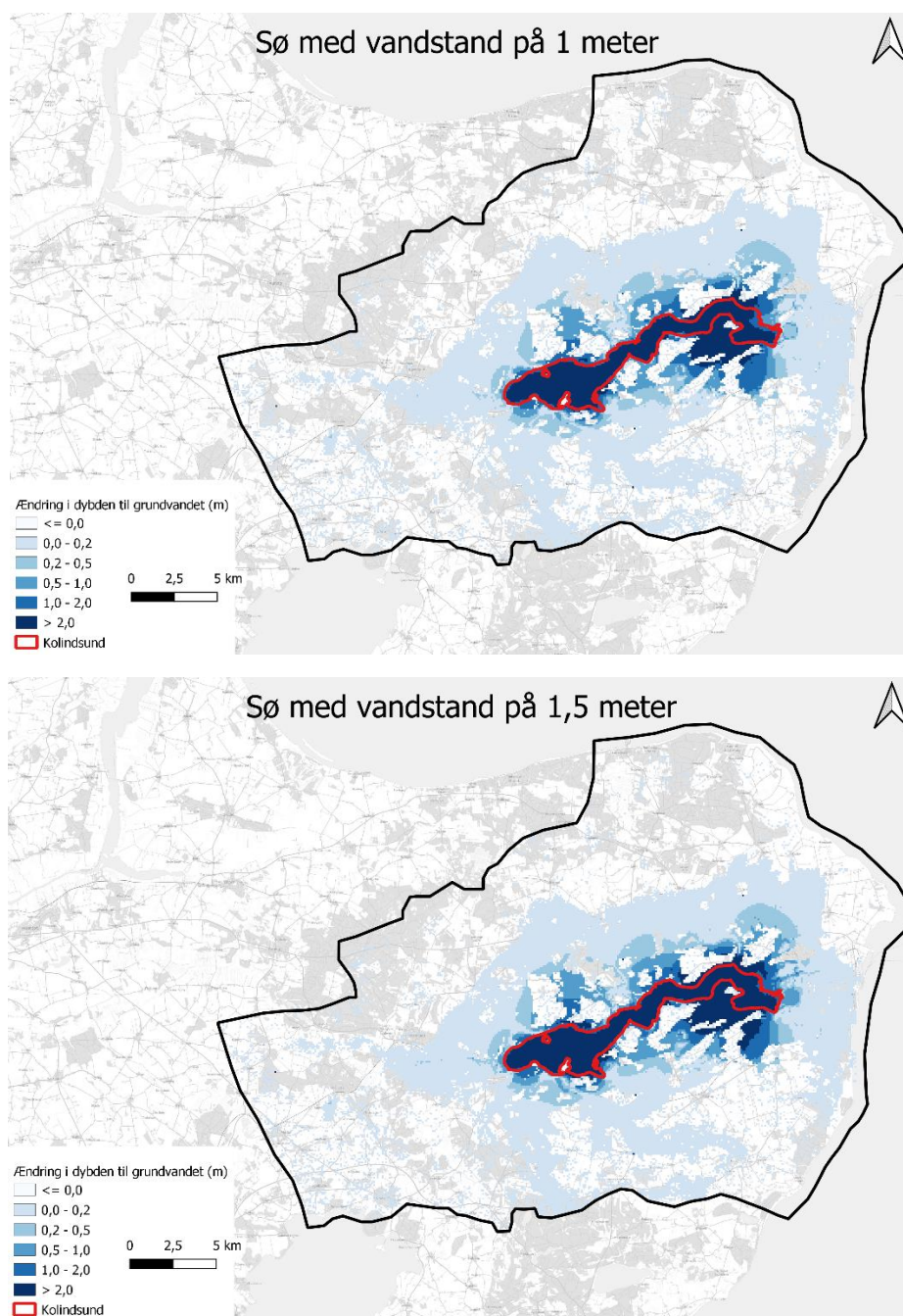
Figur 9.19 Ændring i grundvandsspejlet ved etablering af en sø med en vandstand på 1 m (øverst) og 1,5 m (nederst). Grundvandsstanden vil blive påvirket over 5 km fra søen.
