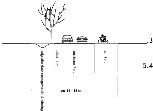
Vejprofil
