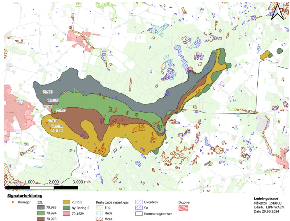
Figur 7.3. Beskyttet natur omkring kildepladsen i Løvenholmskoven. Indvindingsoplande for de seks borerer på kildepladsen ved indvinding af op til 1,5 mill. m 3 råvand om året. Indvindingsoplandene er tillagt en buffer på 100 m.
