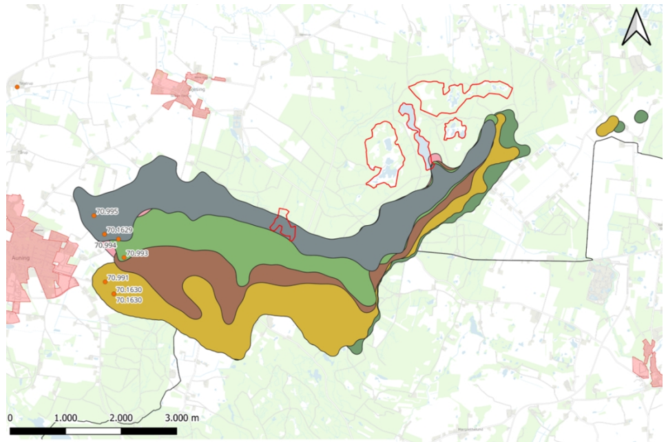
Figur 7.4. Indvindingsoplande for de seks boringer på kildepladsen ved indvinding af op til 1,5 mill. m 3 råvand om året. Figuren viser endvidere beskyttede Natura 2000-områder i nærheden af kildepladsen. Indvindingsoplandene er tillagt en buffer på 100 m.
