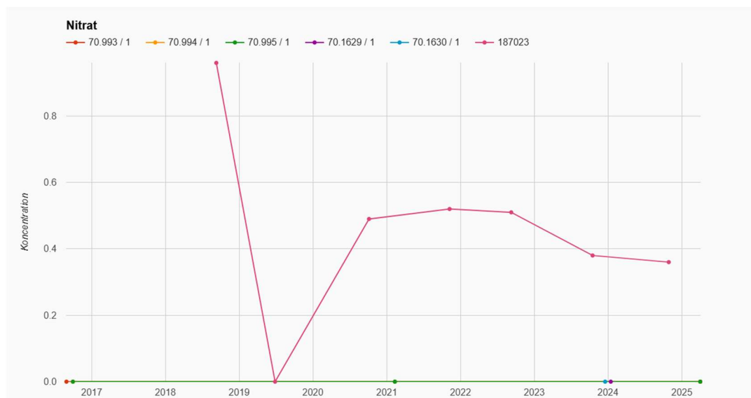
Figur 10.2: Nitratindhold i indvindingsboringerne (DGU nr. 70.991, 70.993, 70.994, 70.995, 70.1629 og 70.1630) og ved afgang fra vandværket ved Løvenholmskoven (anlægs id 187023). Koncentrationen er angivet i mg/l.
